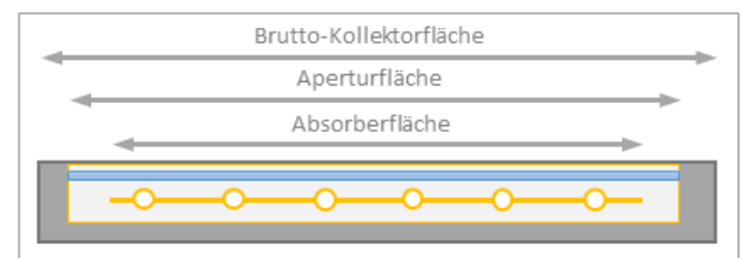
Abbildung 3: Flächenmaße Flachkollektor
