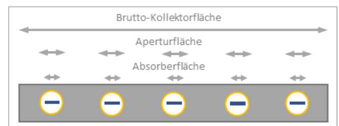
Abbildung 4: Flächenmaße Röhrenkollektor
